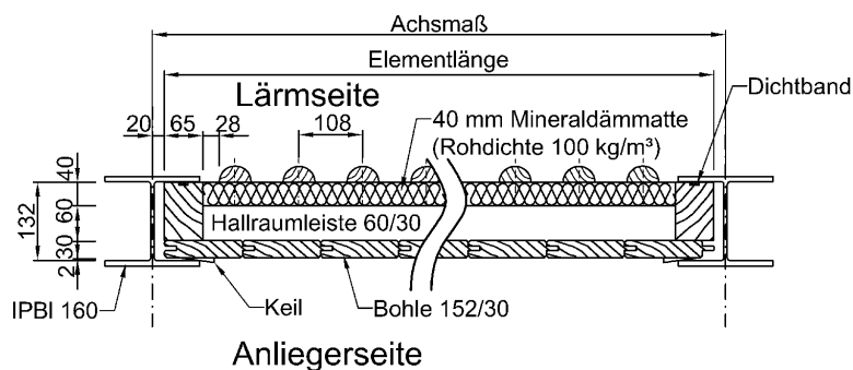
Horizontalschnitt
